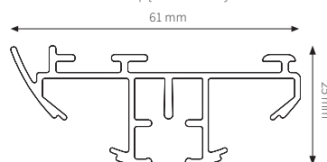
DS-XL Double LED z napędem silnikowym
